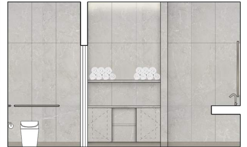
ELEVATION B
