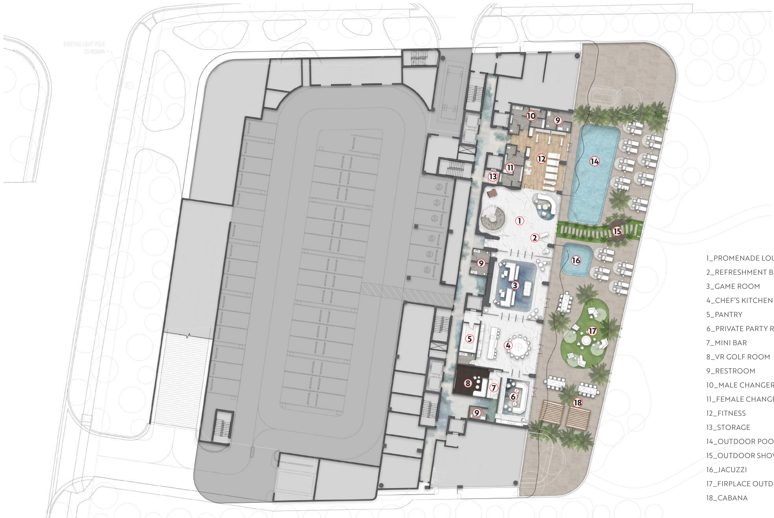
PROMENADE LEVEL(LEVEL 1) PLAN
